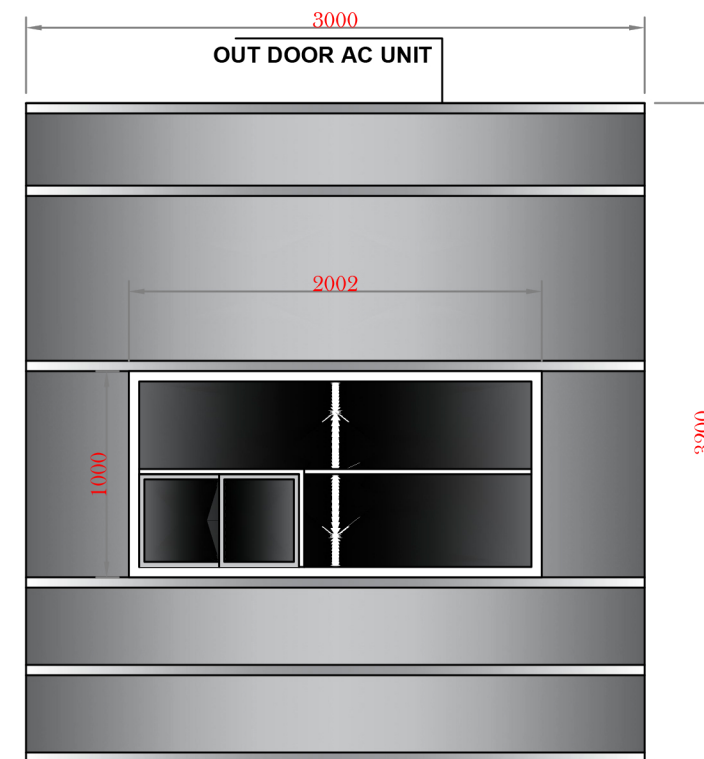
RIGHT ELEVATION
