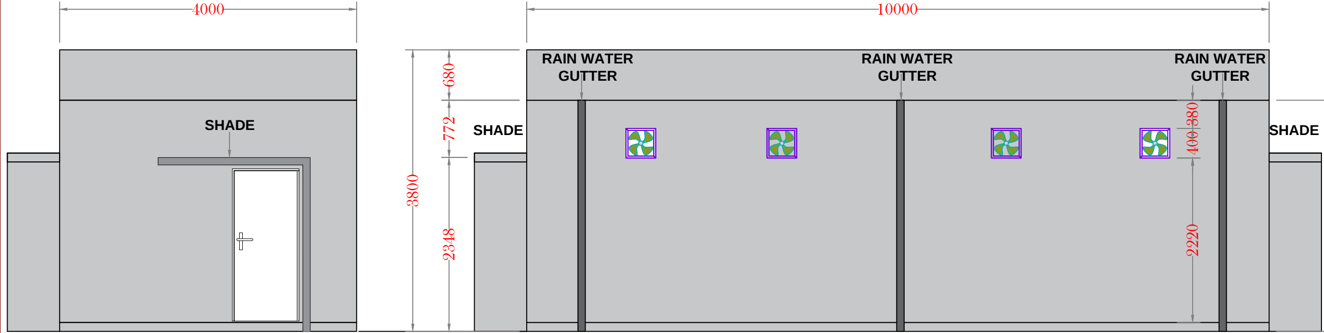
RIGHT ELEVATION
